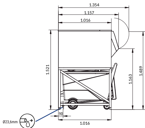
RIGHT SIDE VIEW VISTA LATERAL DERECHA
