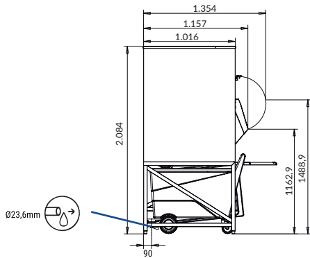
RIGHT SIDE VIEW VISTA LATERALE DESTRA
