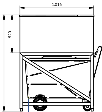
RIGHT SIDE VIEW VISTA LATERAL DERECHA
