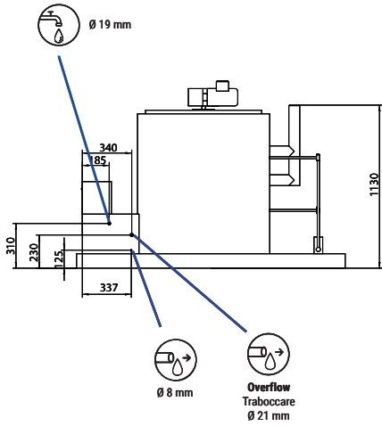
RIGHT SIDE VIEW VISTA LATERALE DESTRA
