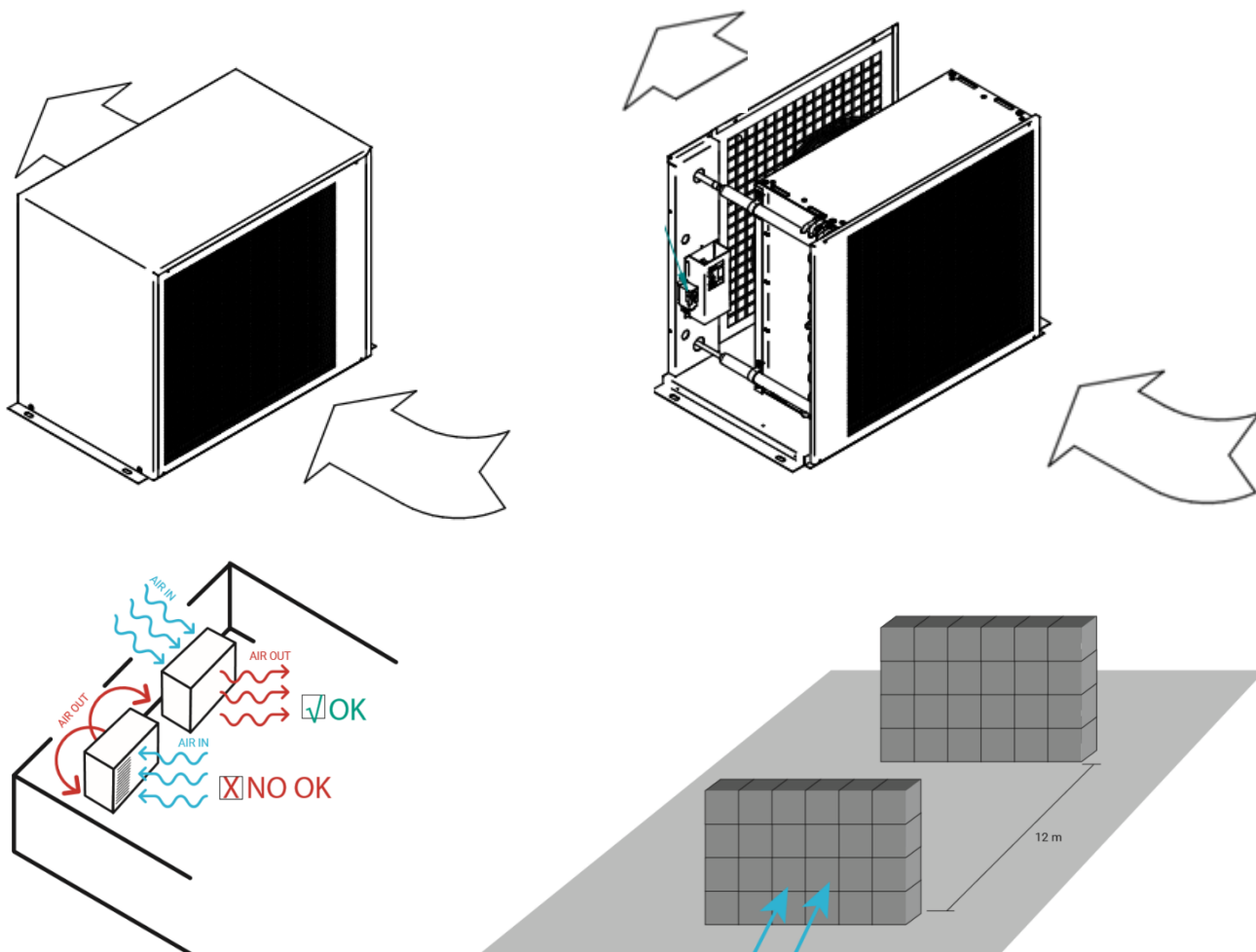
Direzione principale del vento
