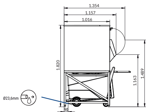
RIGHT SIDE VIEW VISTA LATERAL DERECHA
